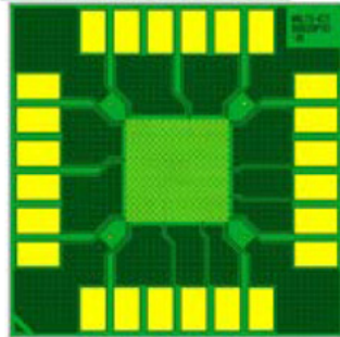
【KIT 01A 120P(S)-10】
