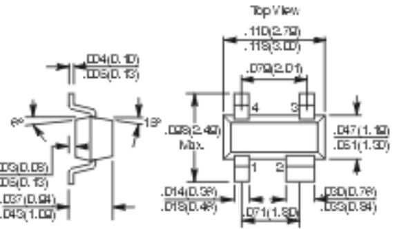
SOT143
