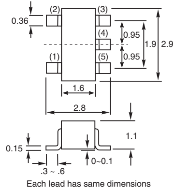
SOT25
