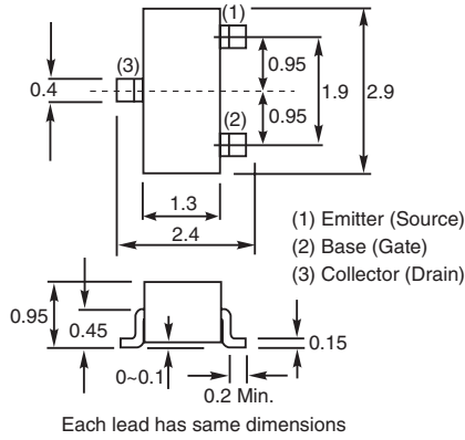
SOT23
