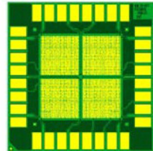
【KIT FC120(S) (2 × 2)】
