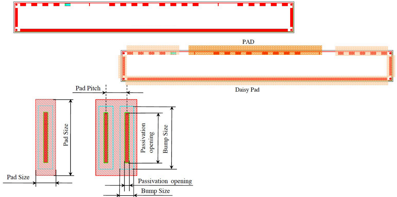
(Daisy Pad)
