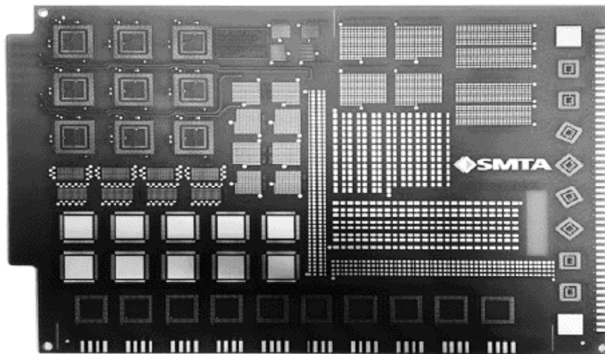
SMTA-H Kit
