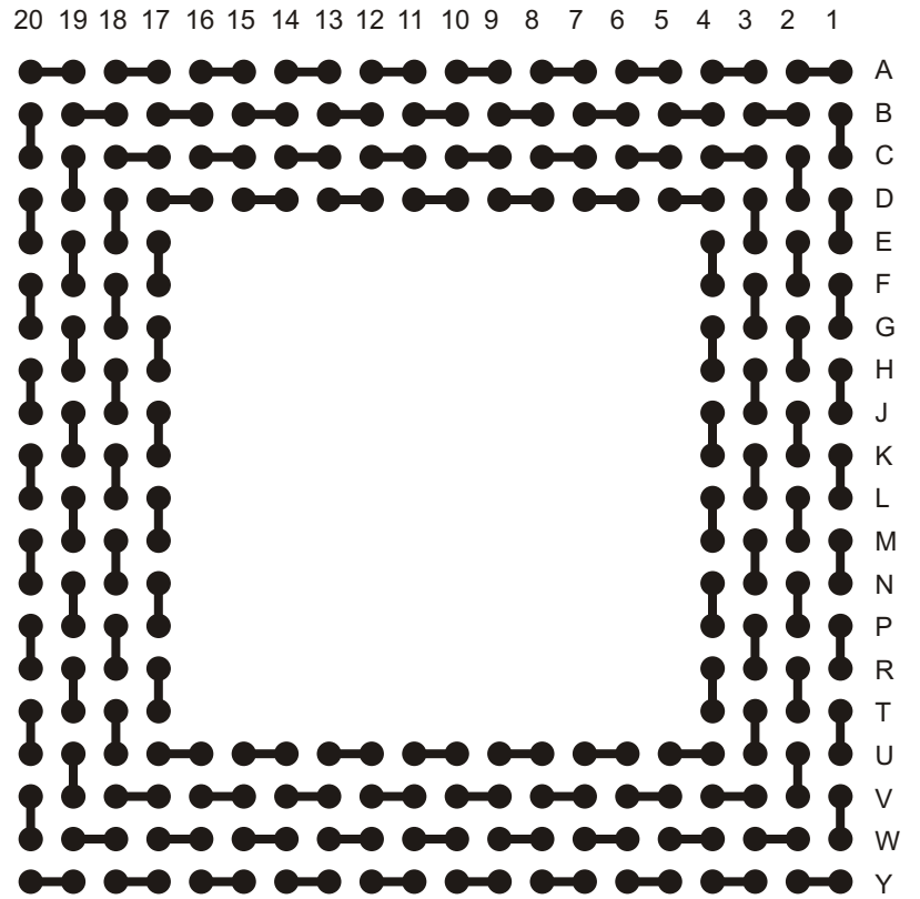
A-PBGA256-1.27mm-27mm
