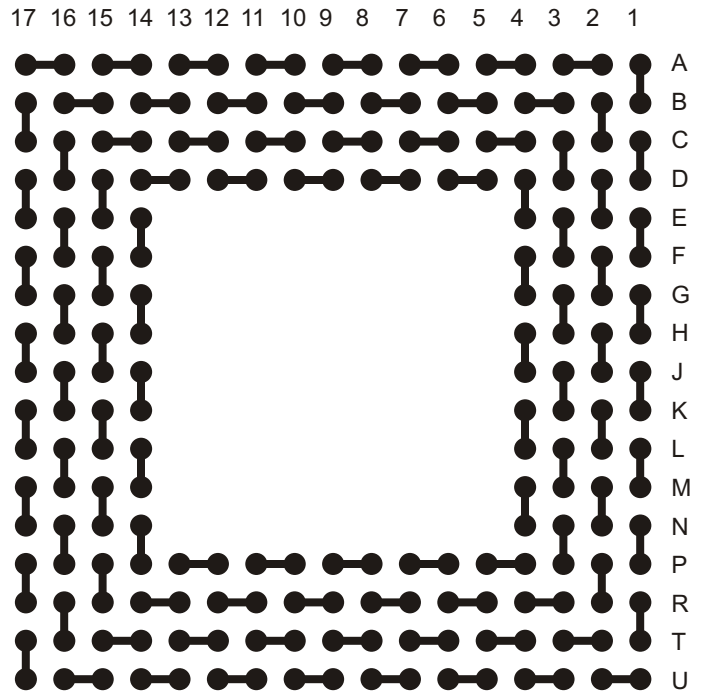
A-CTBGA208-.8mm-15mm-DC
